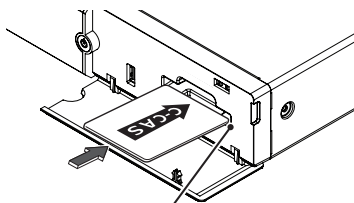
C-CASカード挿入口
